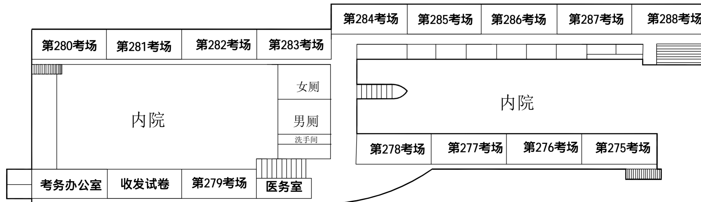
一层平面图
